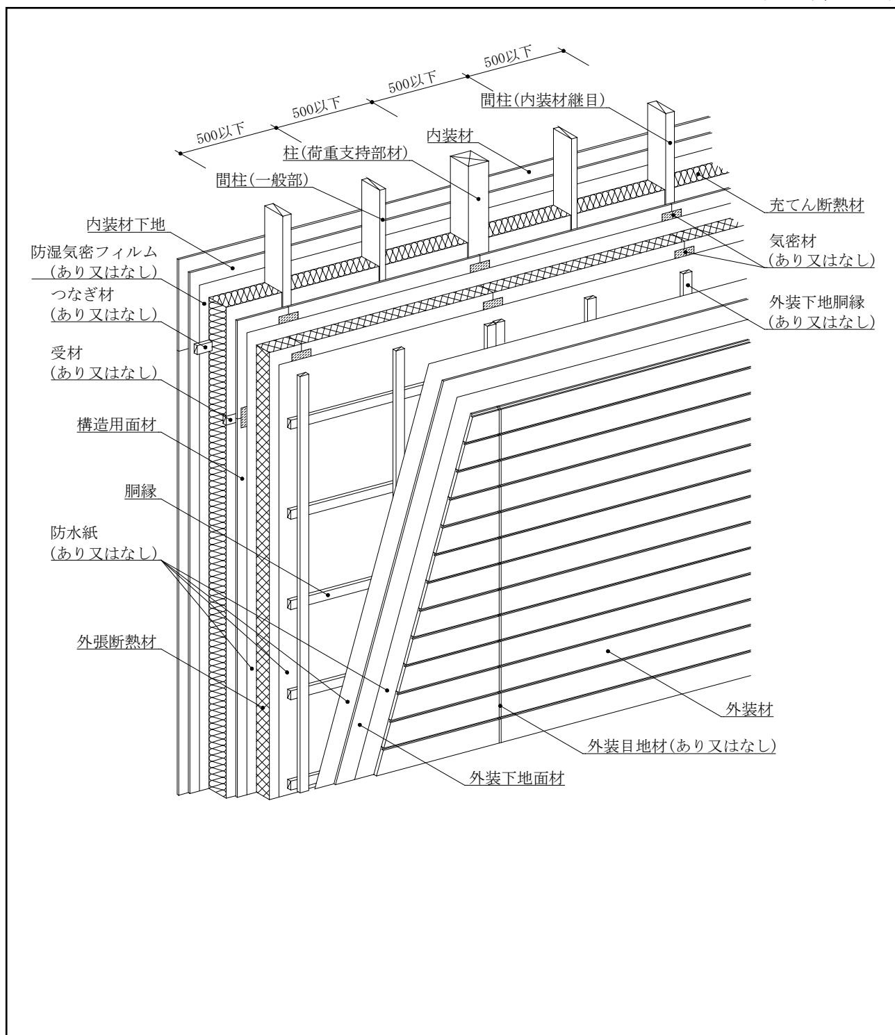
図3 構造説明図
