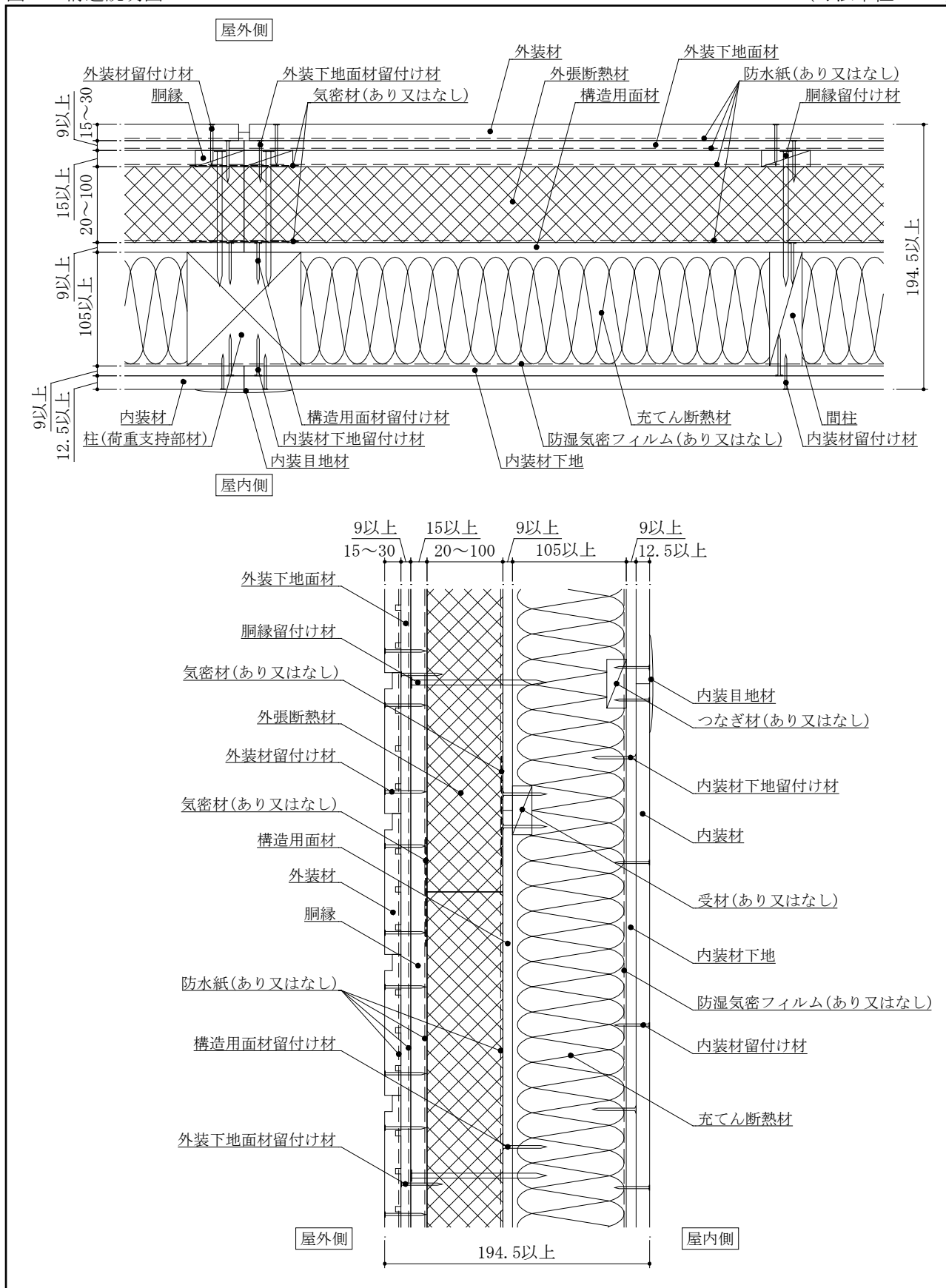
図2 構造説明図
