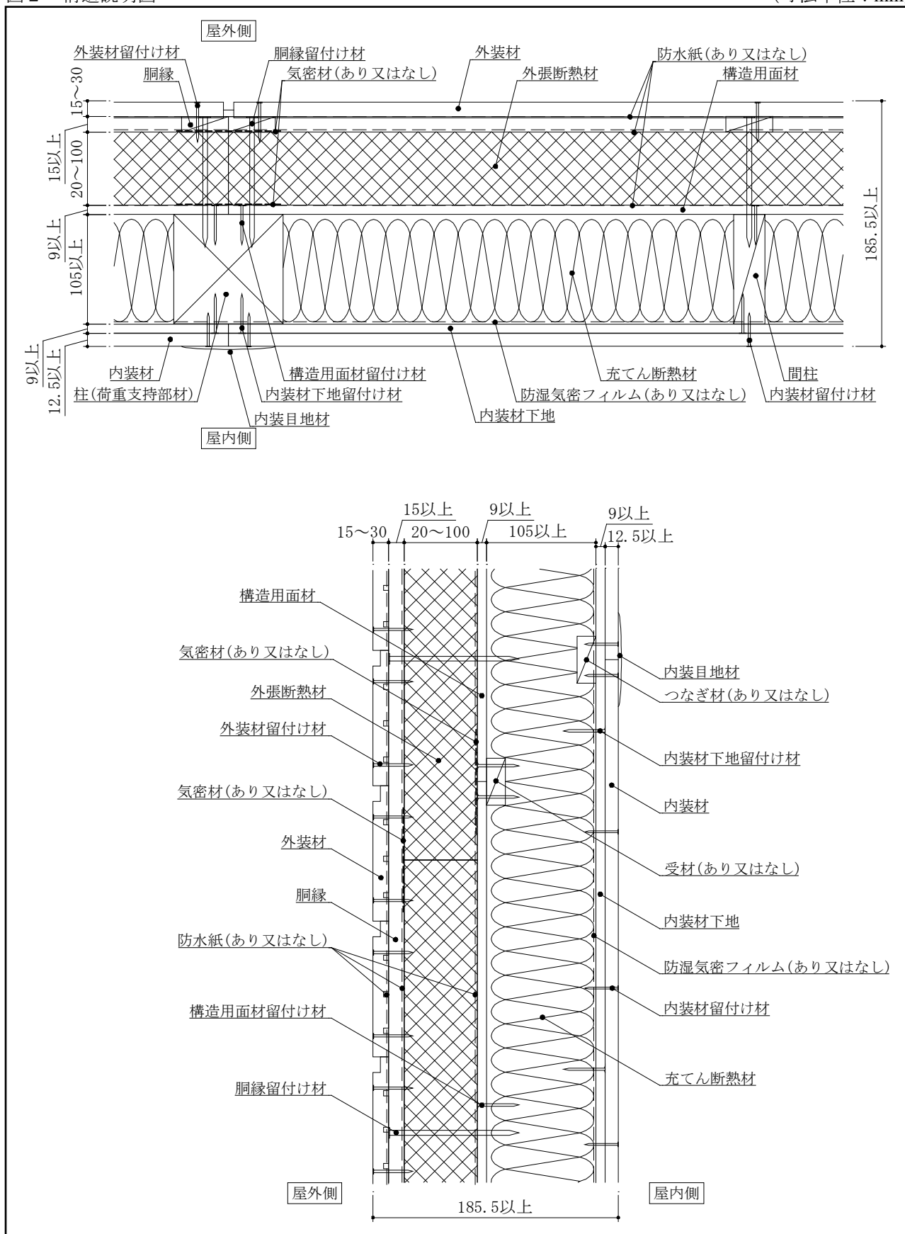
図2 構造説明図
