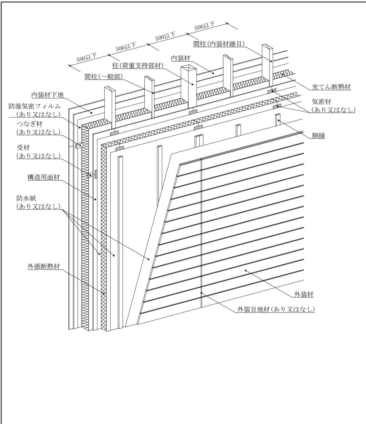
図 1 構造説明図
