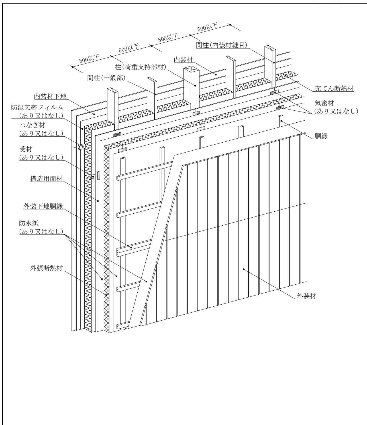
図7 構造説明図
