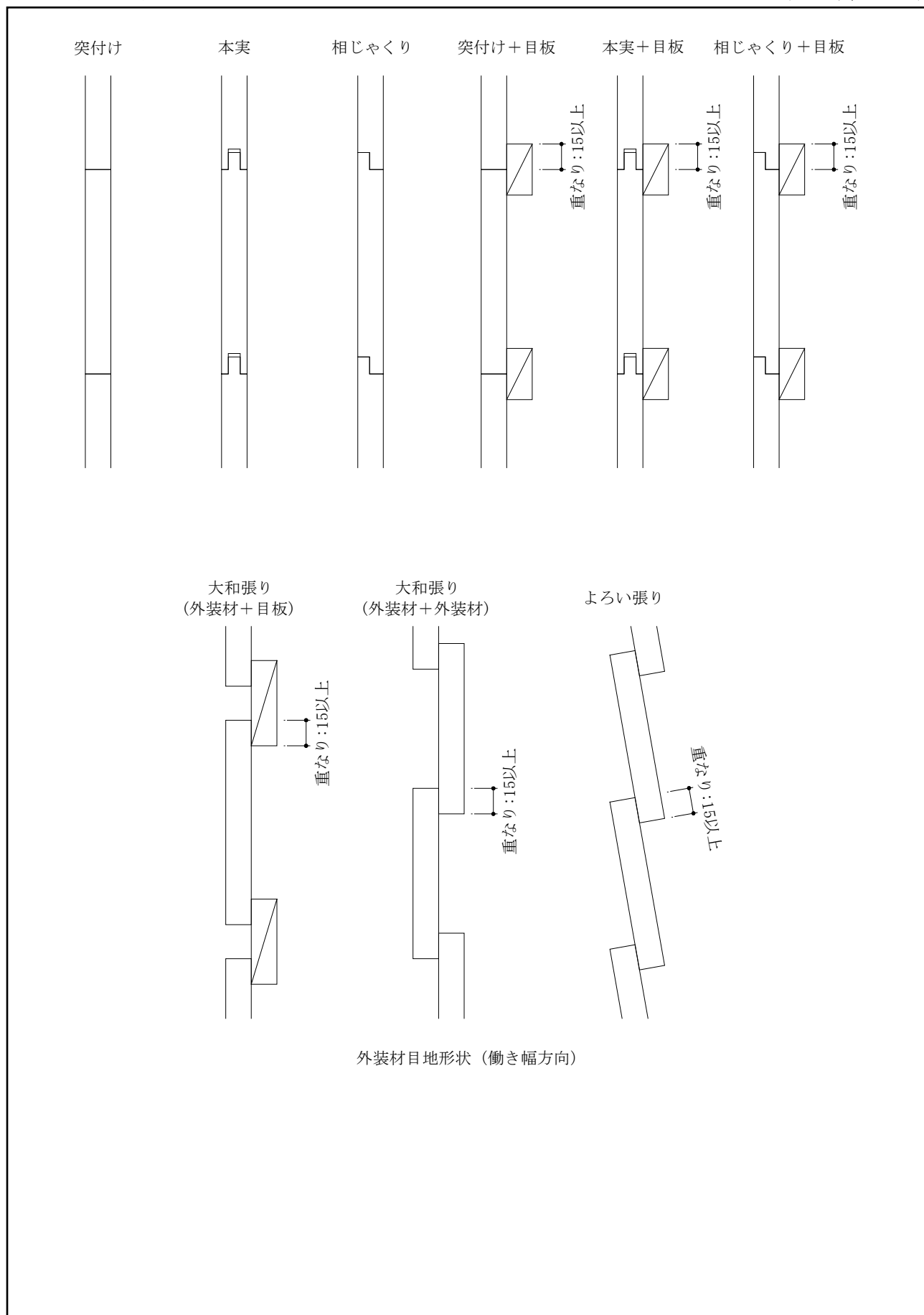
図9 構造説明図
