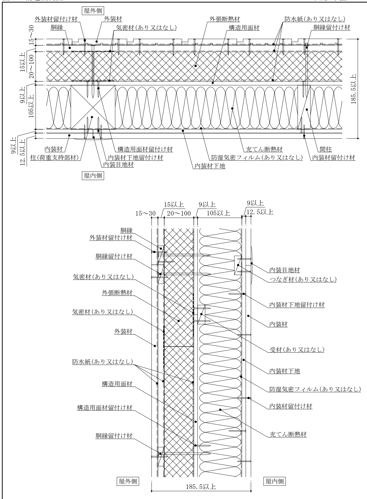
図6 構造説明図
