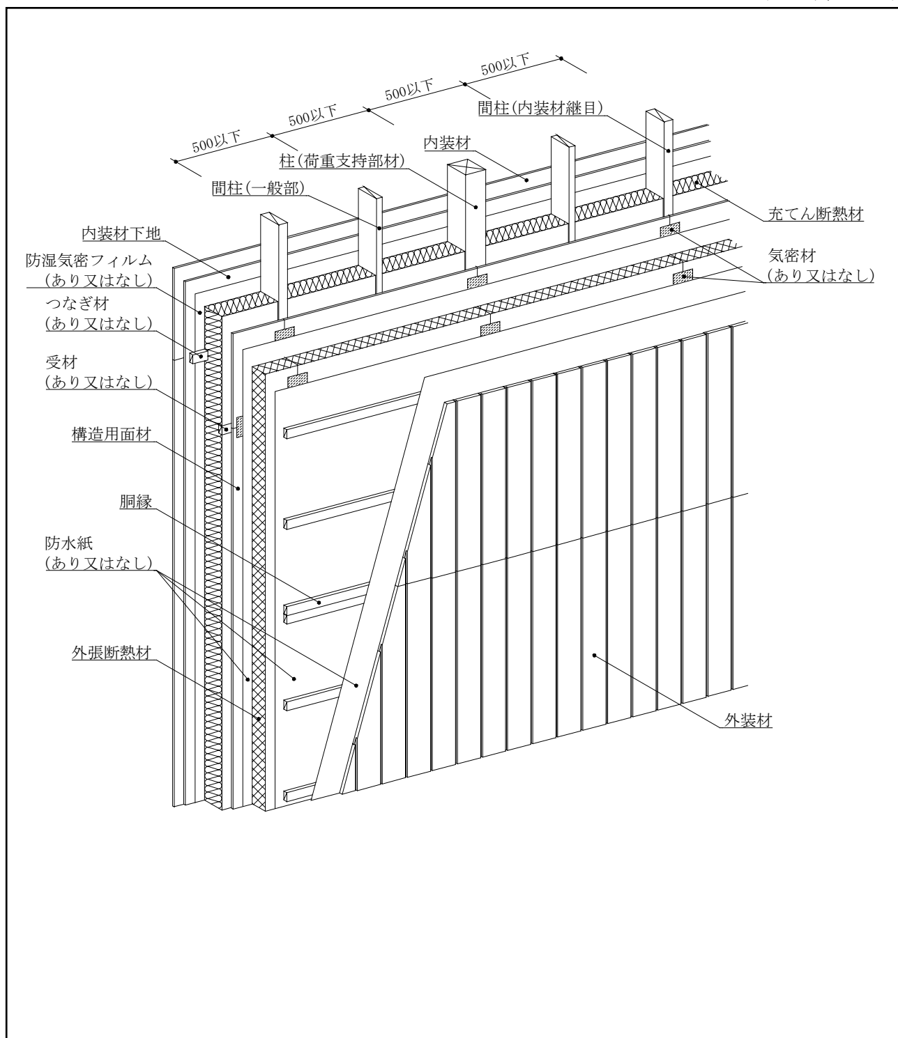
図5 構造説明図
