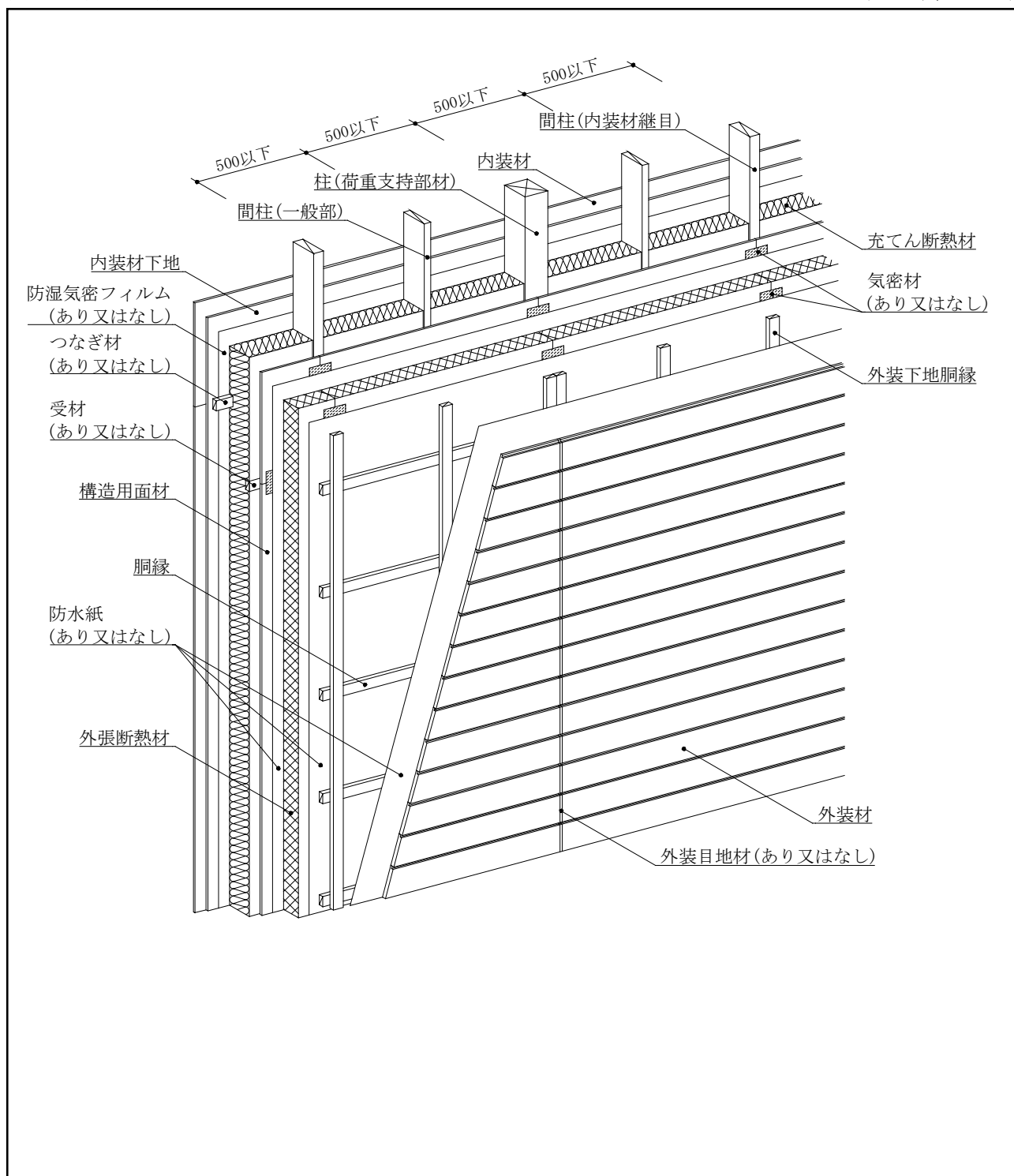
図3 構造説明図
