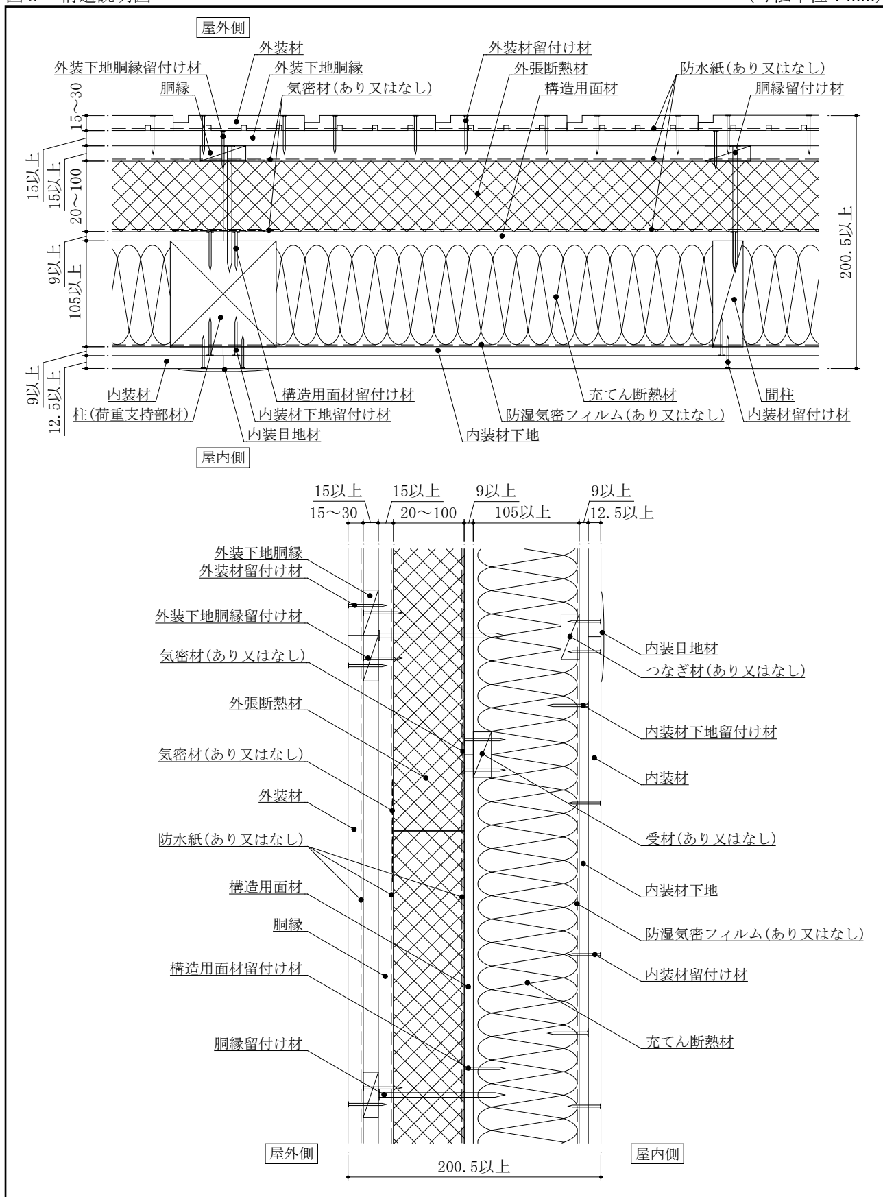
図8 構造説明図
