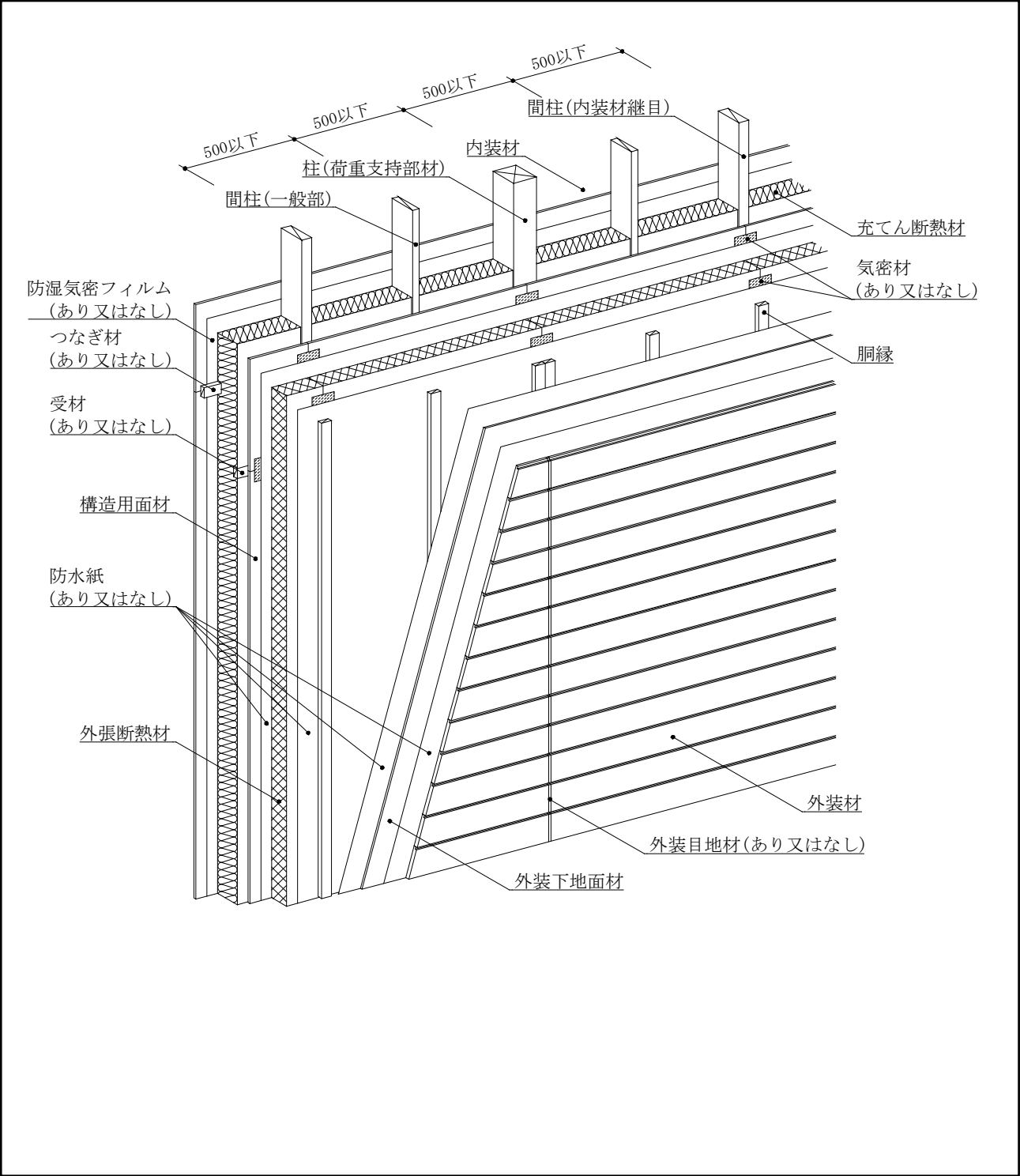
図1 構造説明図 (寸法単位：mm)
