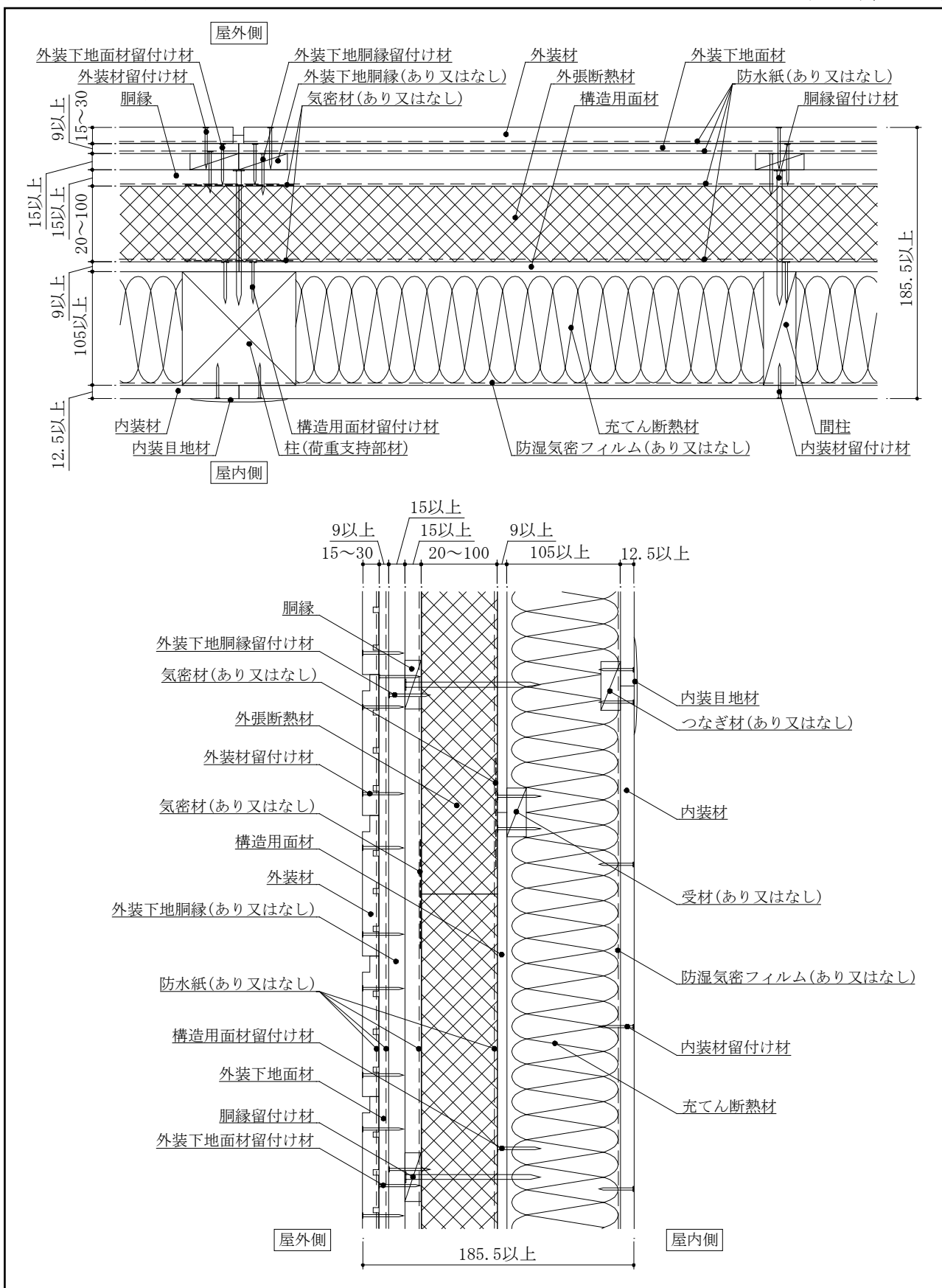
図4 構造説明図
