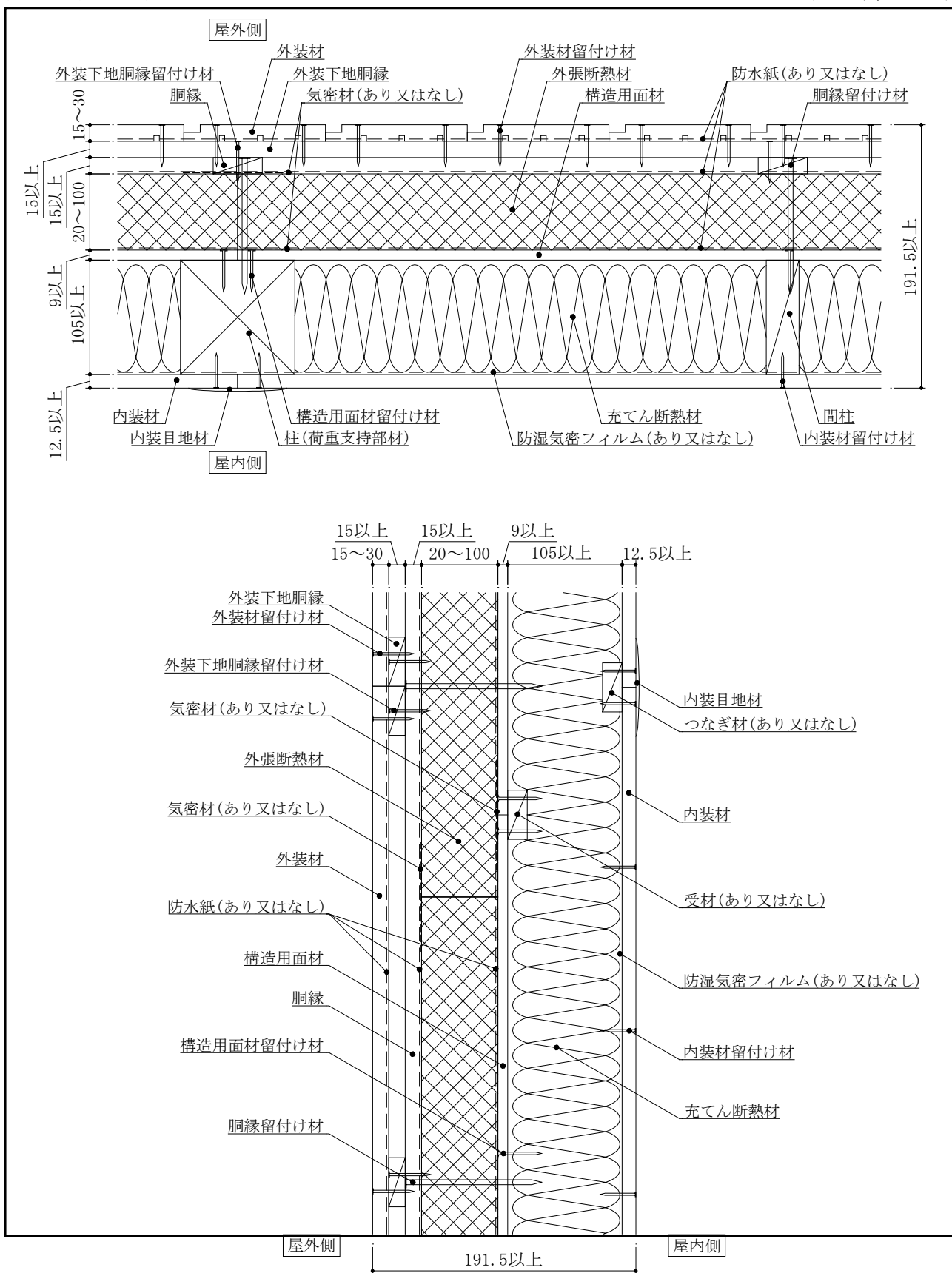
図8 構造説明図
