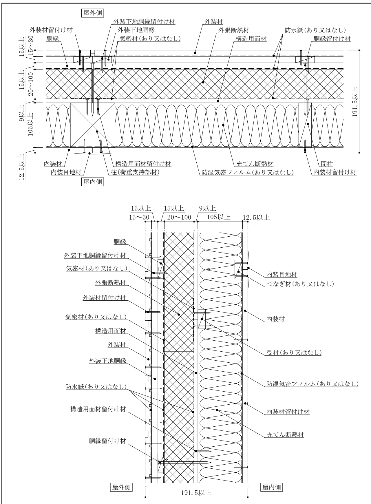
図4 構造説明図
