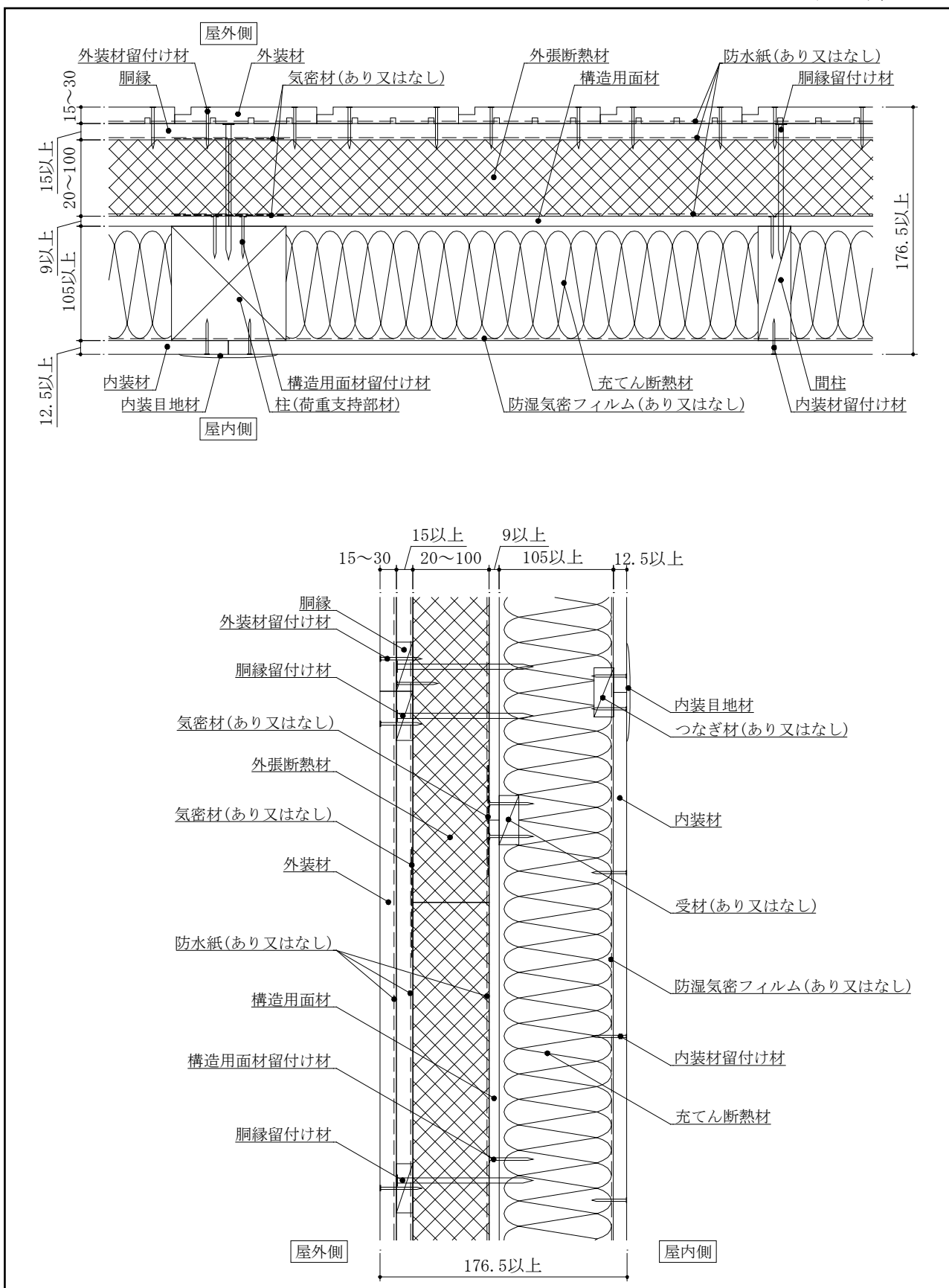
図6 構造説明図
